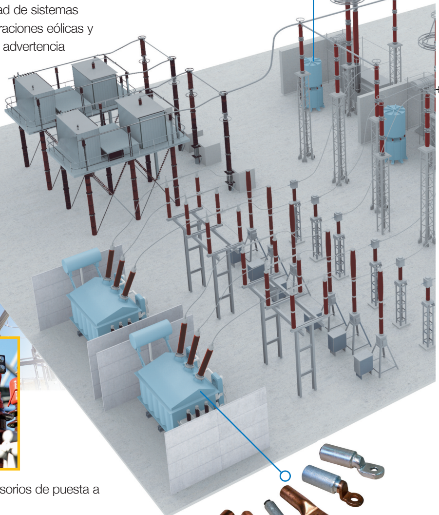
Terminales específicos para subestaciones
