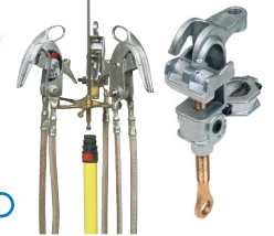
Sistema de puesta a tierra y en cortocircuito para MT
